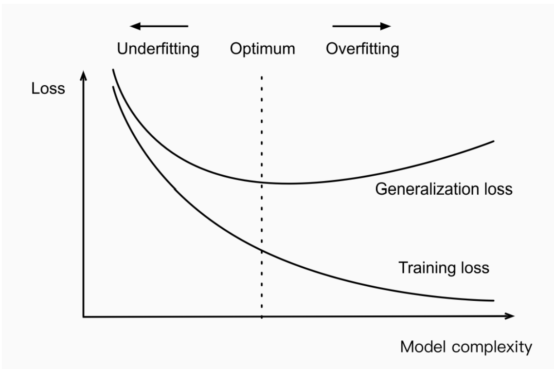
Underfitting und Overfitting vs. Modell-Komplexität.
