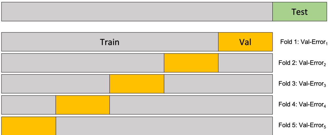
Skizze der n -fold cross-validation für n = 5
